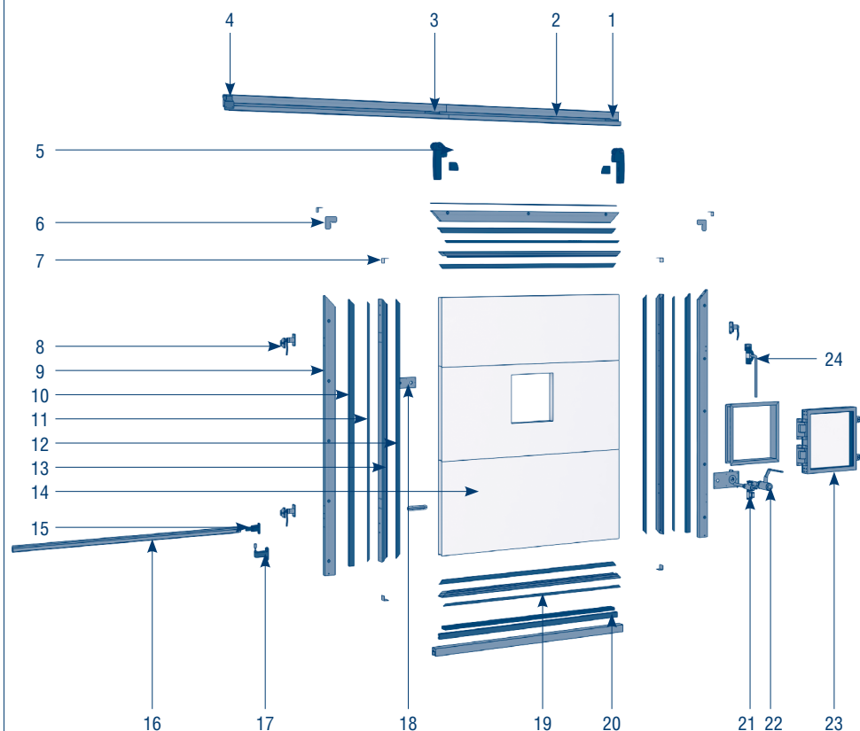
Рис. 1. Разнесенный вид
